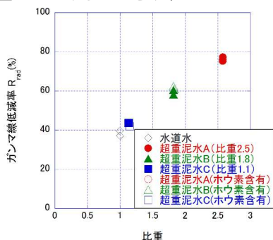
図 4 ガンマ線低減率と比重の関係
