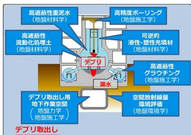
図-1 原子炉周辺における地盤工学の貢献可能性
